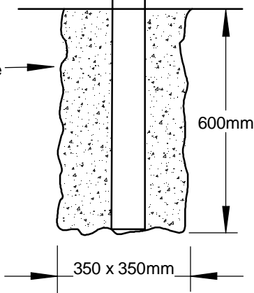
ELEVATION
